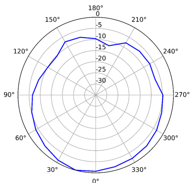
2.4 GHz (Vertical)
