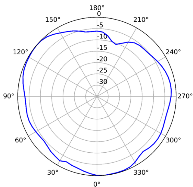
2.4 GHz (Horizontal)
