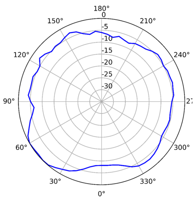
5 GHz (Horizontal)
