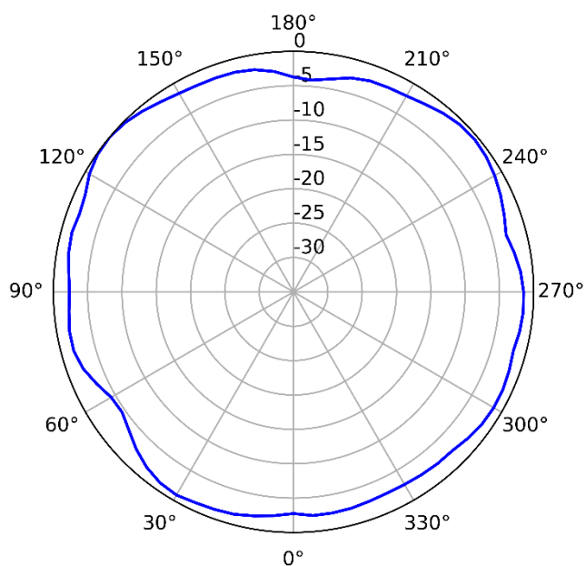
2.4 GHz (horizontal)
